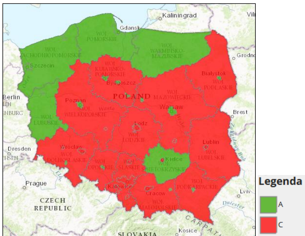
Rycina 8. Stan jakości powietrza w Polsce w 2015 roku - pył PM 2,5
