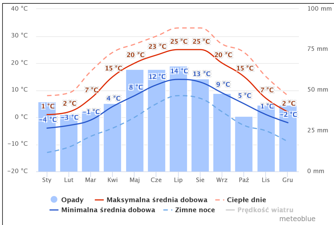
Rycina 5. Średni przebieg temperatury i opadów atmosferycznych w Gminie Kolbiel
