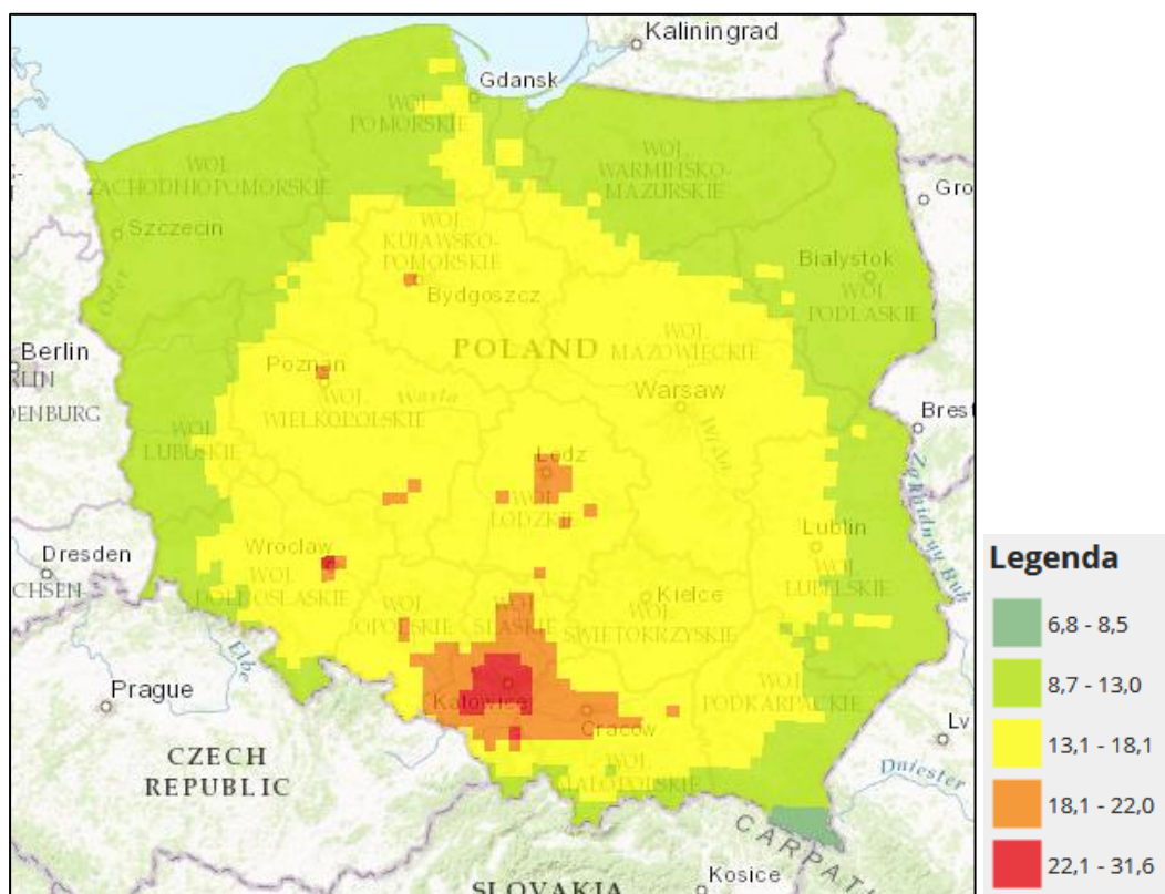
Rycina 9. Prognoza stanu jakości powietrza na rok 2020- pył PM 2,5
