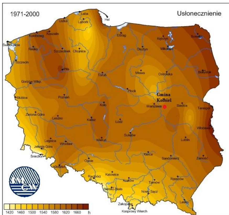
Rycina 4. Średnie roczne wartości usłonecznienia w latach 1971-2000
