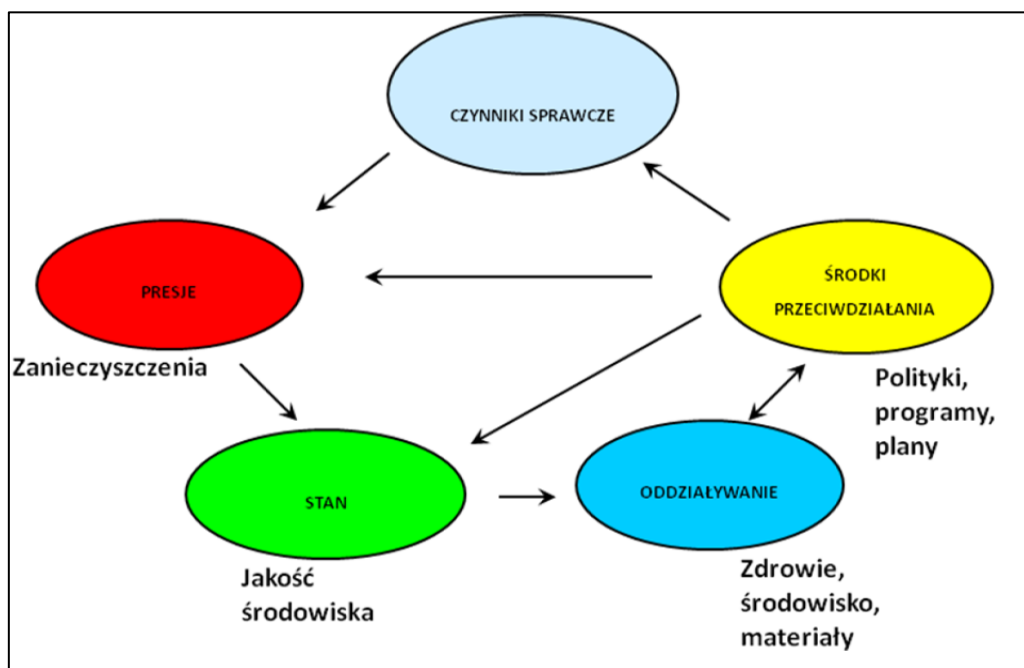
Rycina 22. Model D-P-S-I-R w ochronie środowiska
