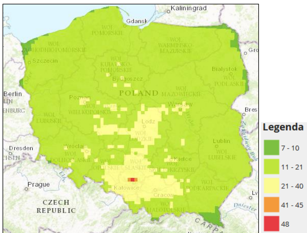
Rycina 11. Prognoza stanu jakości powietrza w 2020 roku- pył PM 10
